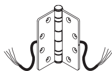
TRANSFERENCIA DE ENERGÍA BISAGRA PLANA INTERMEDIA
